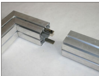
UNION PERFIL AL ANGULO
